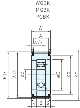
中心軸承型 (1PCS軸承時)
